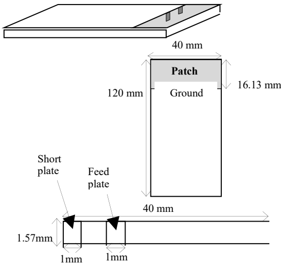
Fig. 1. PIFA Antenna
